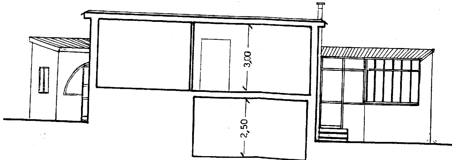
SEZ. A A'
